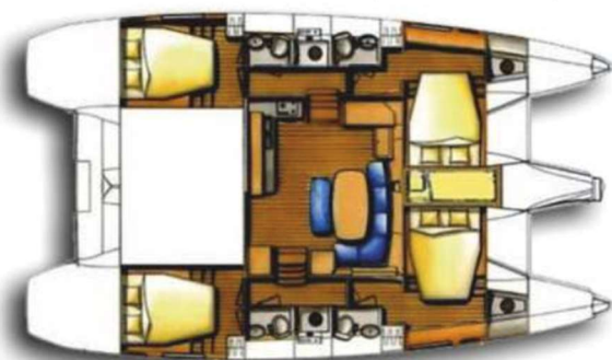
LAGOON 421 L = 12,61 m B = 7,50 m
