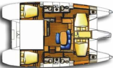
LAGOON 421 L = 12,61 m B = 7,50 m
